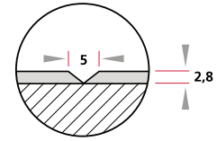
Birdsmouth joint Bec de moineau
